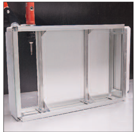
Scheletro cassonetto
